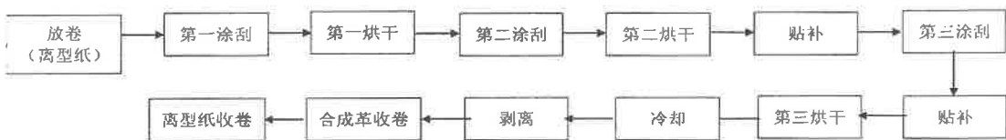
图 33-4 聚氨酯干法工艺生产工艺流程图
