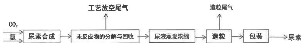
图 25-5 尿素生产工艺流程图
