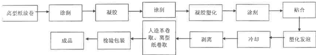
图 33-2 聚氯乙烯离型纸法生产工艺流程图
